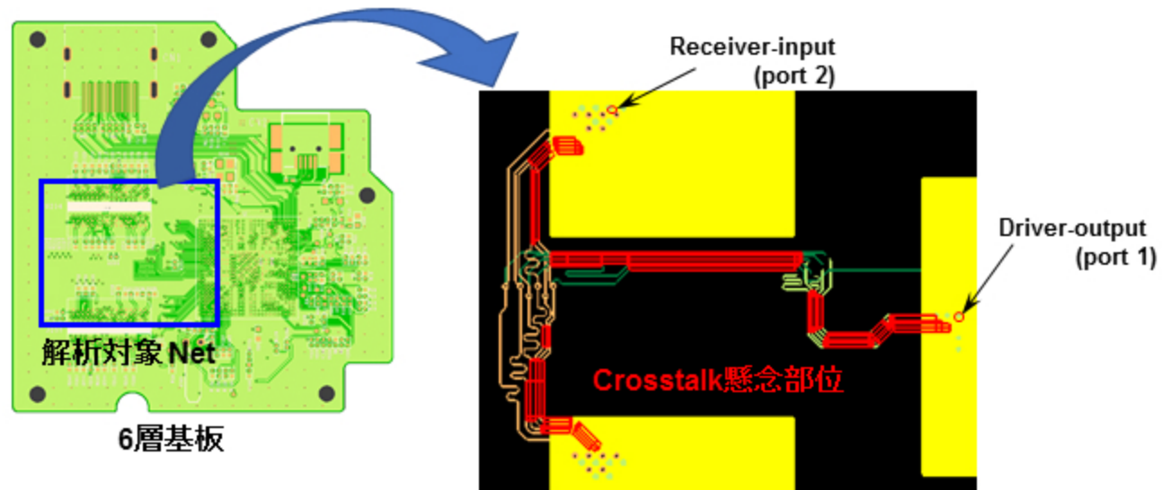
ビクティム + 5系統のアグレッサー
