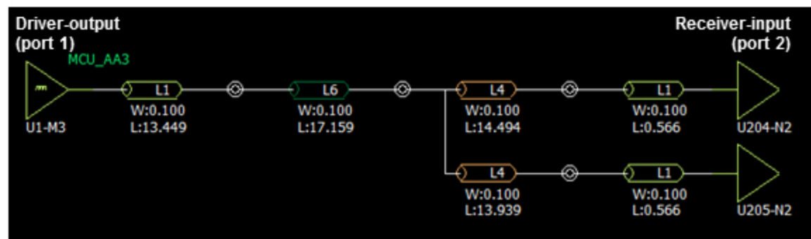
ビクティムの Netトポロジー
